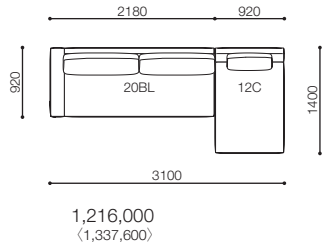
SNA-20(B)L · 12C
