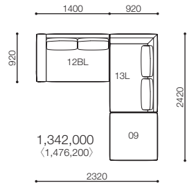
SNA-12(B)L · 13L · 09
