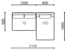
SNA-12・12C
