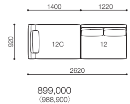
SNA-12C · 12
