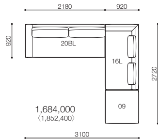
SNA-20(B)L · 16L · 09
