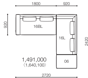
SNA-16(B)L · 16L · 06
