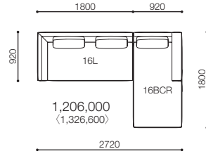
SNA-16(B)L · 16(B)CR
