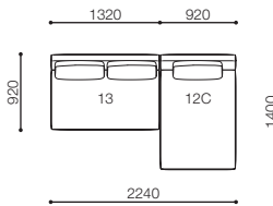
SNA-13・12C
