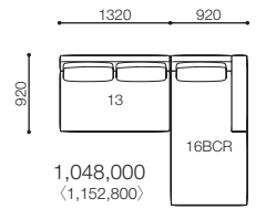
SNA-13・16(B)CR
