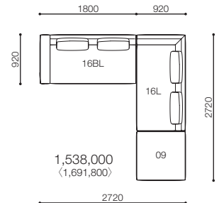
SNA-16(B)L · 16L · 09
