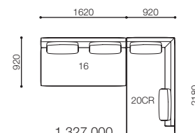
SNA-16・20CR
