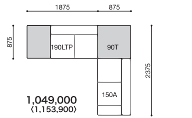
MIO-190LTP · 90T · 150A
