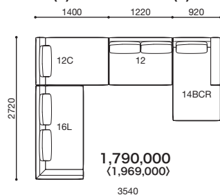
SNA-16(B)L・12C・12・14(B)CR
