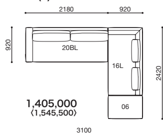
SNA-20(B)L・16L・06
