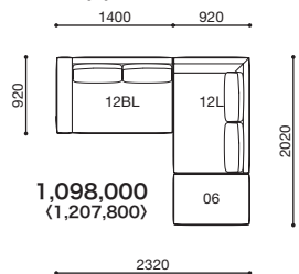
SNA-12(B)L・12L・06
