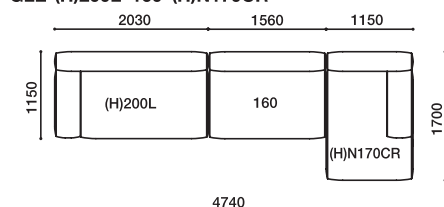
GLE-(H)200L·160·(H)N170CR
