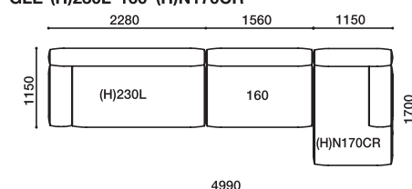
GLE-(H)230L·160·(H)N170CR
