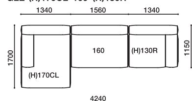
GLE-(H)170CL·160·(H)130R
