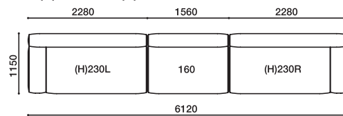
GLE-(H)230L·160·(H)230R
