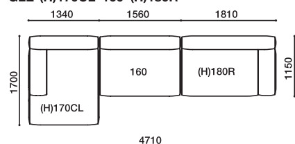
GLE-(H)170CL·160·(H)180R
