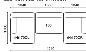
GLE-(H)170CL·160·(H)170CR
