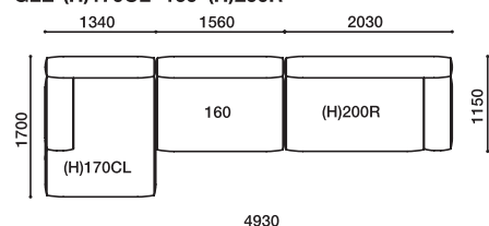
GLE-(H)170CL·160·(H)200R
