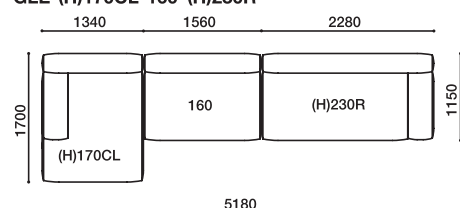
GLE-(H)170CL·160·(H)230R
