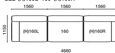
GLE-(H)160L·160·(H)160R
