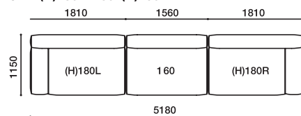
GLE-(H)180L·160·(H)180R
