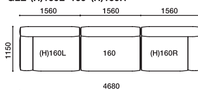
GLE-(H)160L・160・(H)160R
