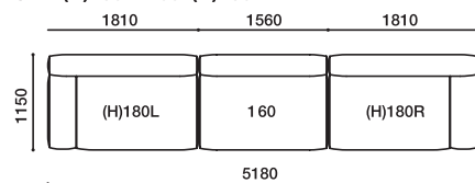
GLE-(H)180L・160・(H)180R
