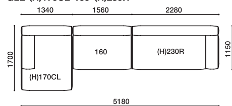
GLE-(H)170CL・160・(H)230R
