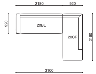
SNA-20(B)L · 20CR
