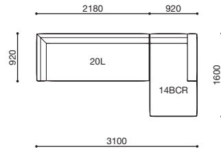
SNA-20(B)L · 14(B)CR
