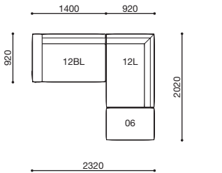
SNA-12(B)L · 12L · 06
