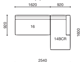
SNA-16 · 14(B)CR
