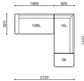
SNA-16(B)L · 16L · 06
