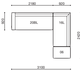
SNA-20(B)L · 16L · 06
