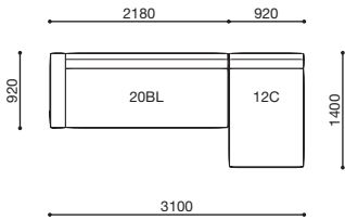
SNA-20(B)L · 12C
