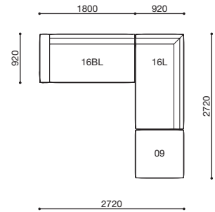
SNA-16(B)L · 16L · 09
